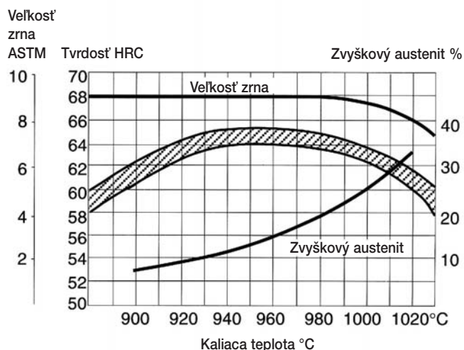
Tvrdosť ako funkcia kaliacej teploty
