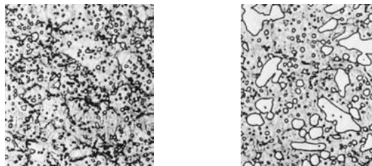
Porovnanie mikroštruktúr RiGOR vs. ledeburická oceľ 1.2080 / 19436
